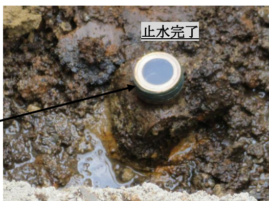
仮本管から個人宅への引き込み接続作業終了
