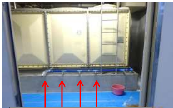
地下貯水槽から飲料水を供給
