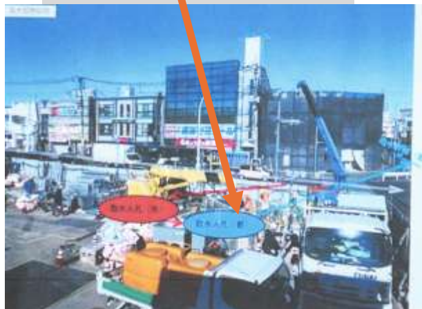
図20；東大和市駅前(立坑)取水人孔
