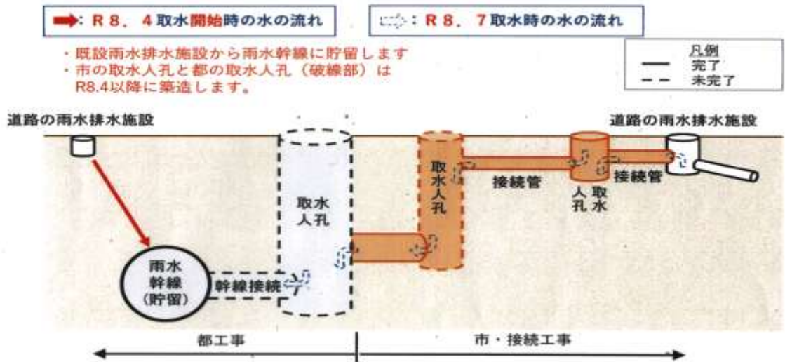
図 1 5 ; 東大和市駅前取水孔の例
