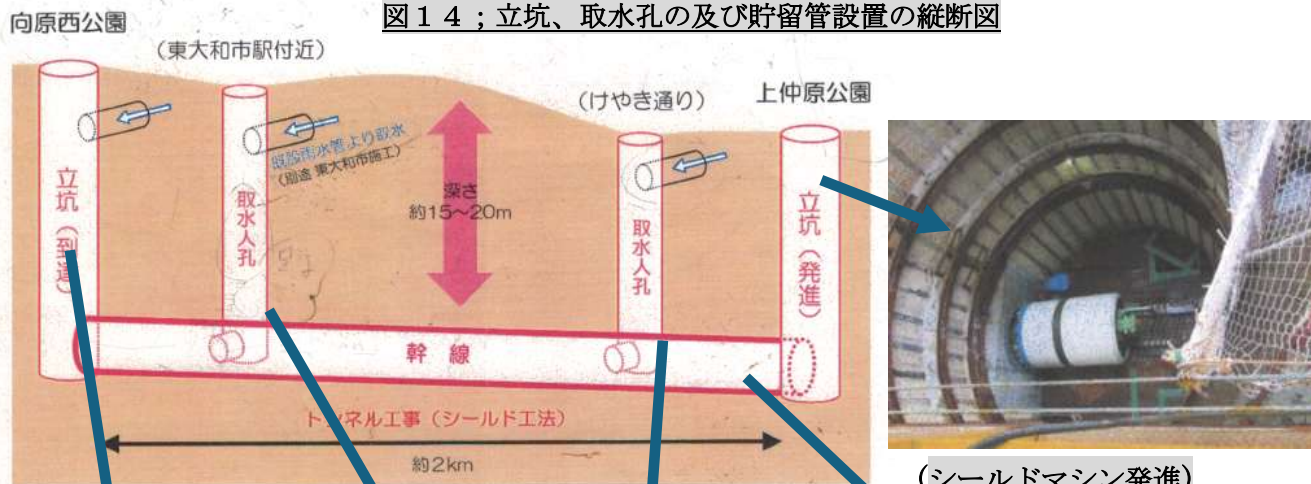
《縦断面図》
